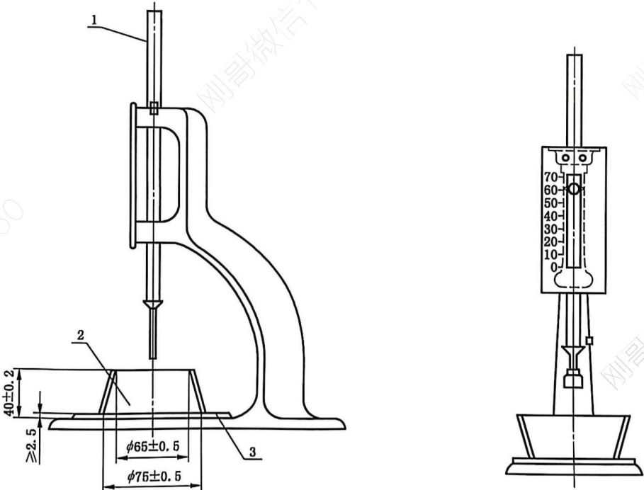
a) 初凝时间测定用试模的侧视图 b) 终凝时间测定时反转试模后的侧视图
