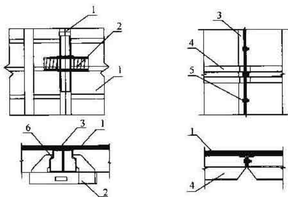
图 1 模板之间的连接
