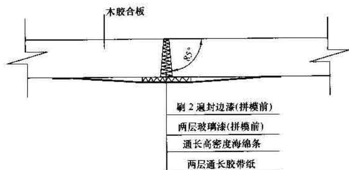
图6 蝉缝的处理
