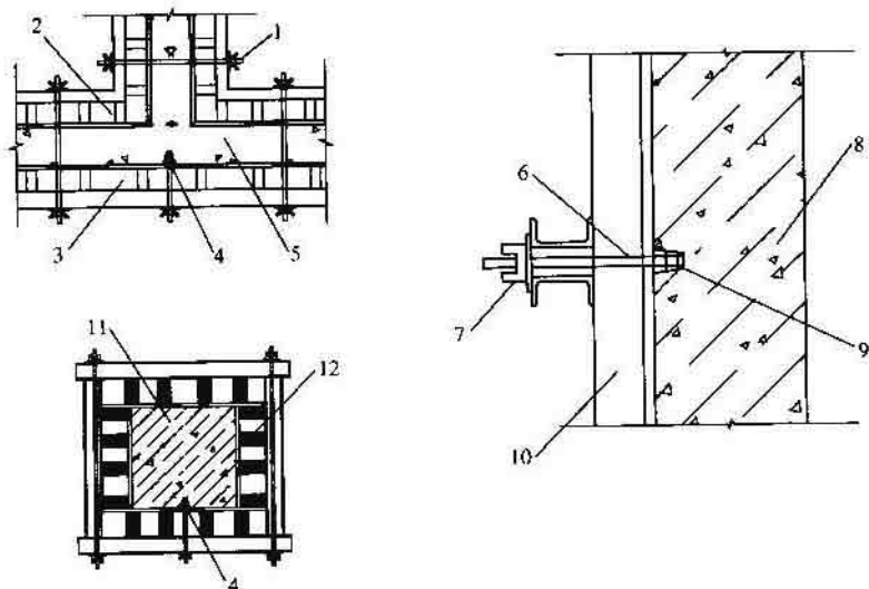
图8 假眼的位置
