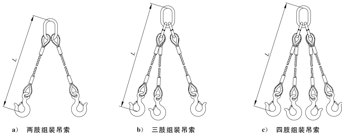
图 2 多肢组装吊索结构
