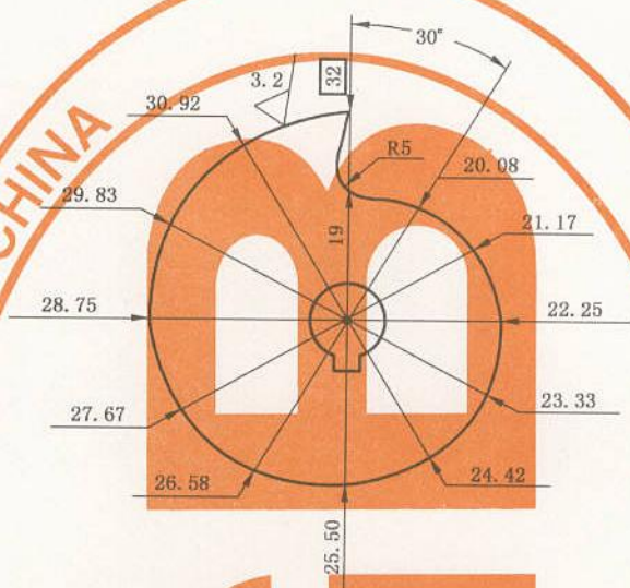
图 A.2 凸轮示意图
