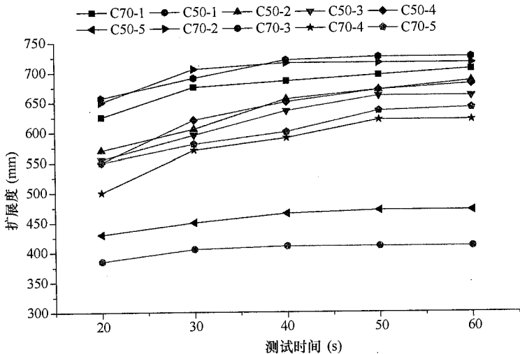
图 4 测试时间对拌合物扩展度的影响
