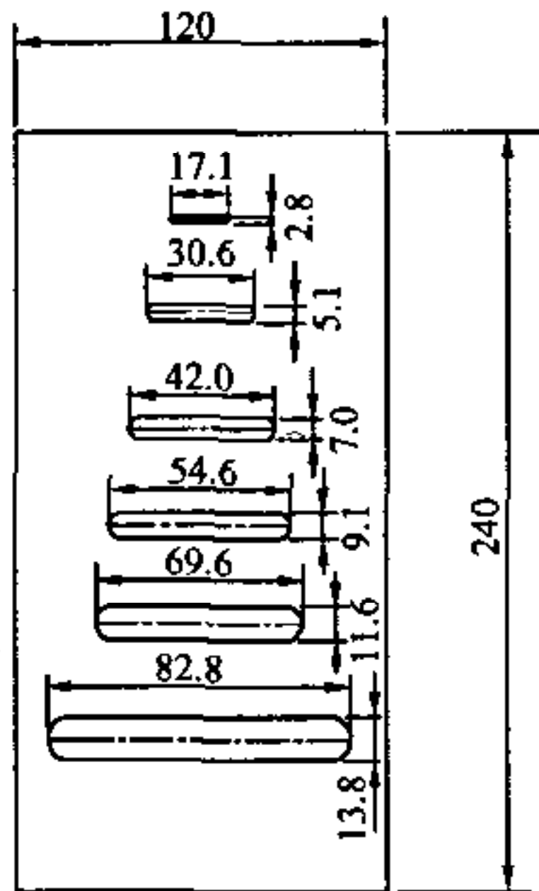
图 7.9.2-2 片状规 准仪 (单位: mm)
