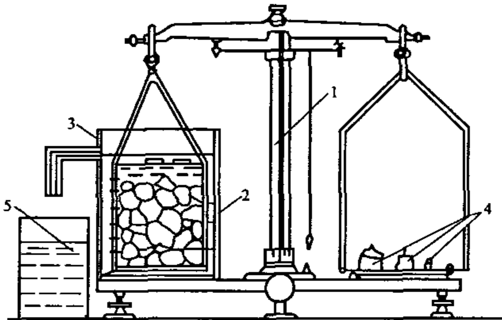
图 7.2.2 液体天平
